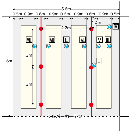
トルコギキョウ1試験区の設計と照度測定点
