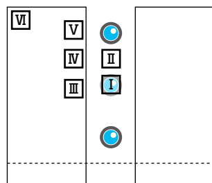
電照光源照度測定点 高さ：ベンチから1.2m
