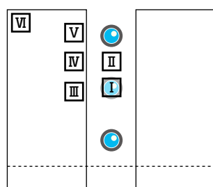
電照光源照度測定点 高さ：地面から1.8m
