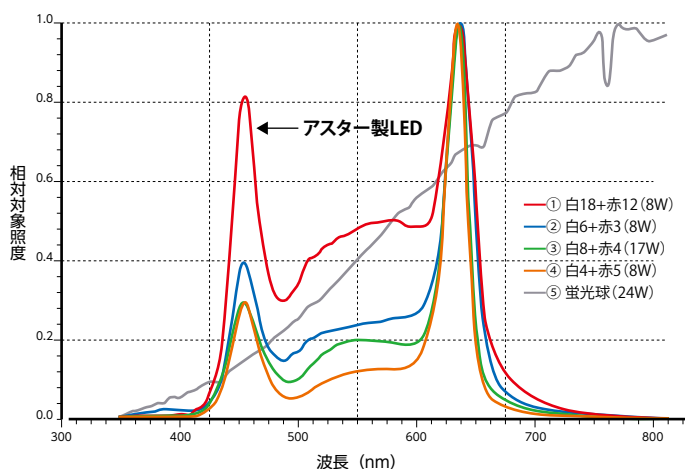
電照菊圃場に設置した電照光源の分光分布
