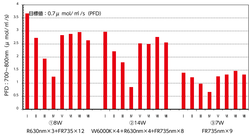
各試験区の照度測定値と仕様充足率
