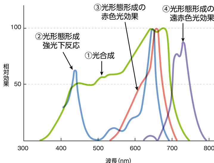
植物の光反応の作用スペクトル (文部科学省より)
