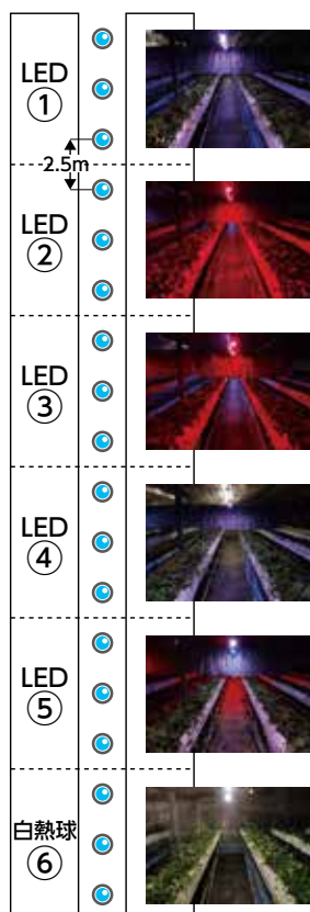
電照光源照度測定点 高さ：ベンチから1.2m
