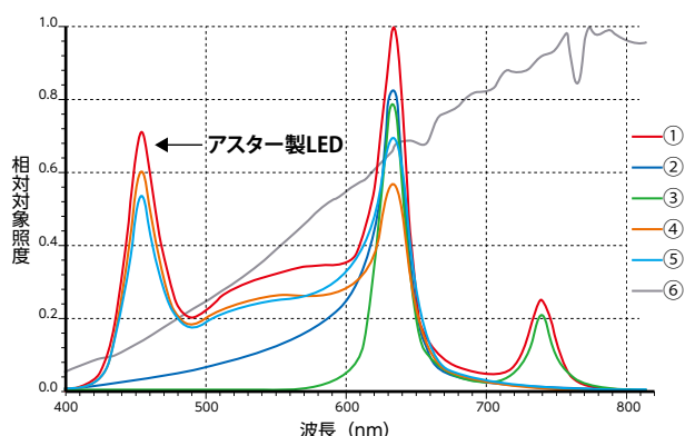
さがほのか電照光源の相対光分布
