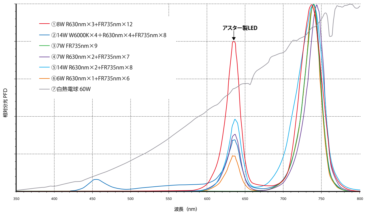
トルコギキョウ圃場各試験区の電照光源の相対分光分布
